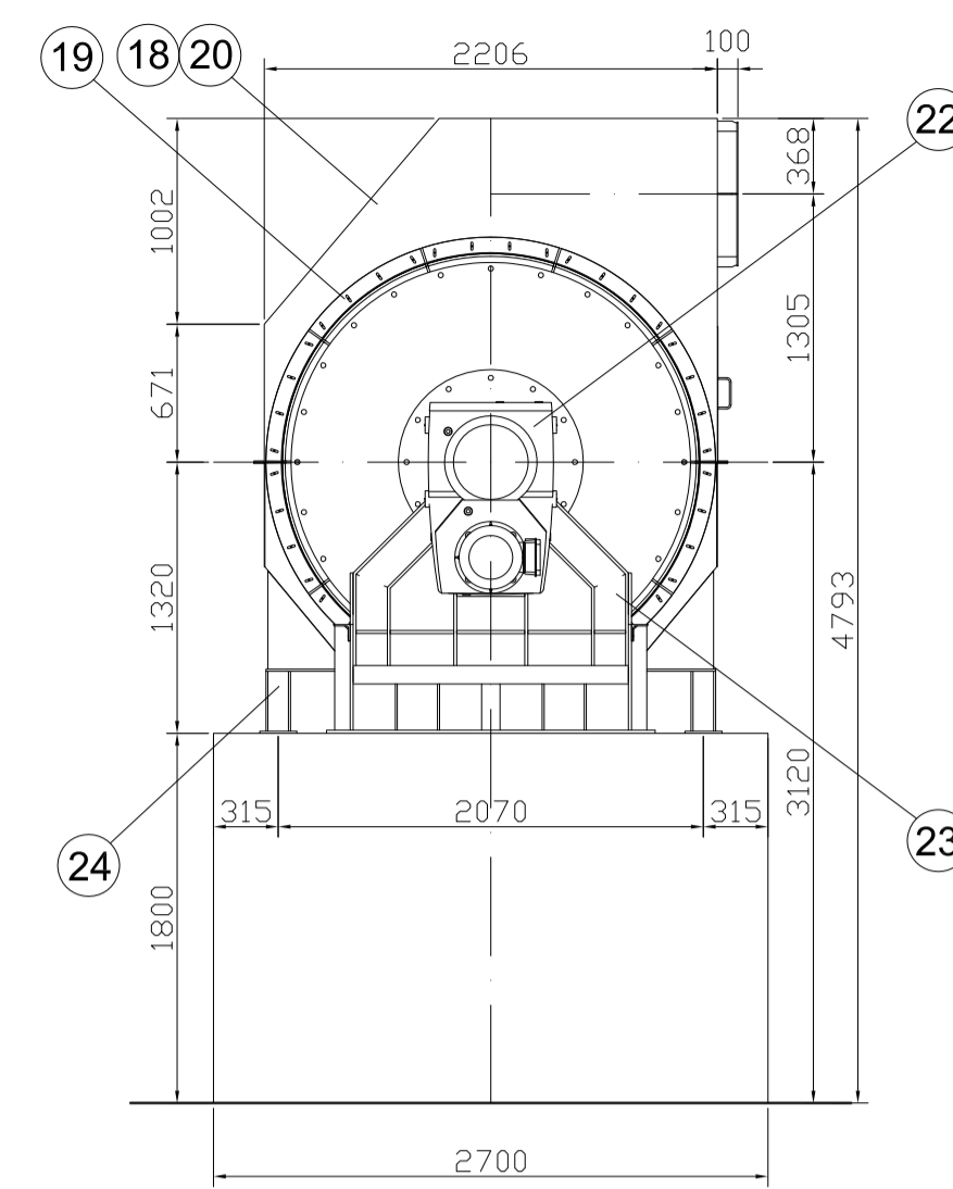
VISTA LATO RIDUTTORE "B-B" 1:40
