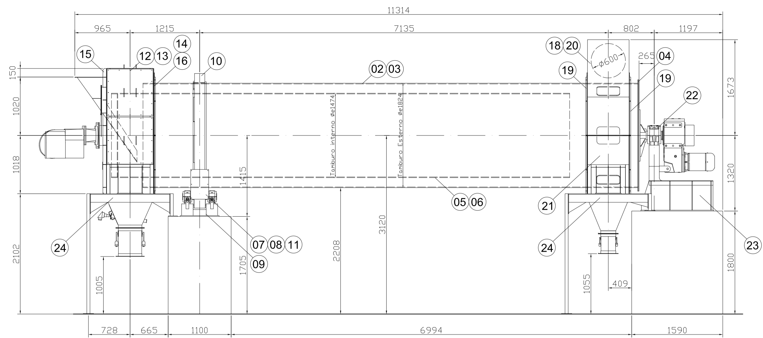
VISTA LATERALE "A-A" 1:40
