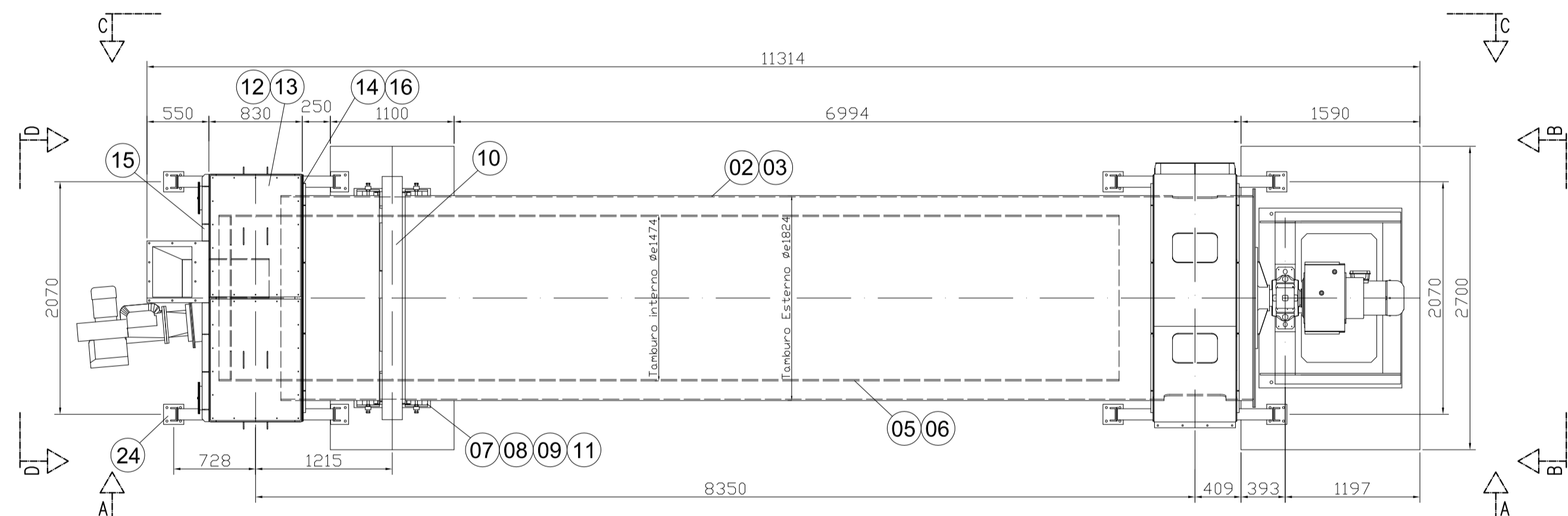
VISTA DALL'ALTO 1:40
