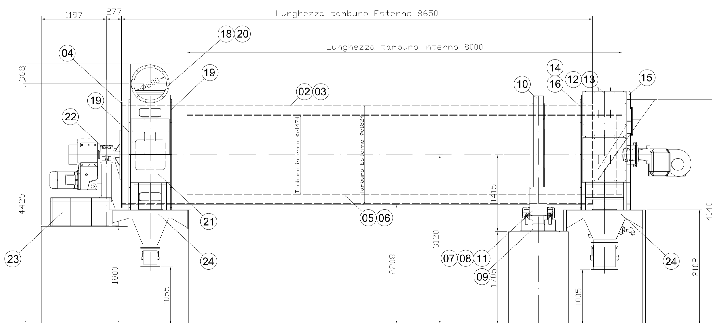
VISTA LATERALE "C-C" 1:40
